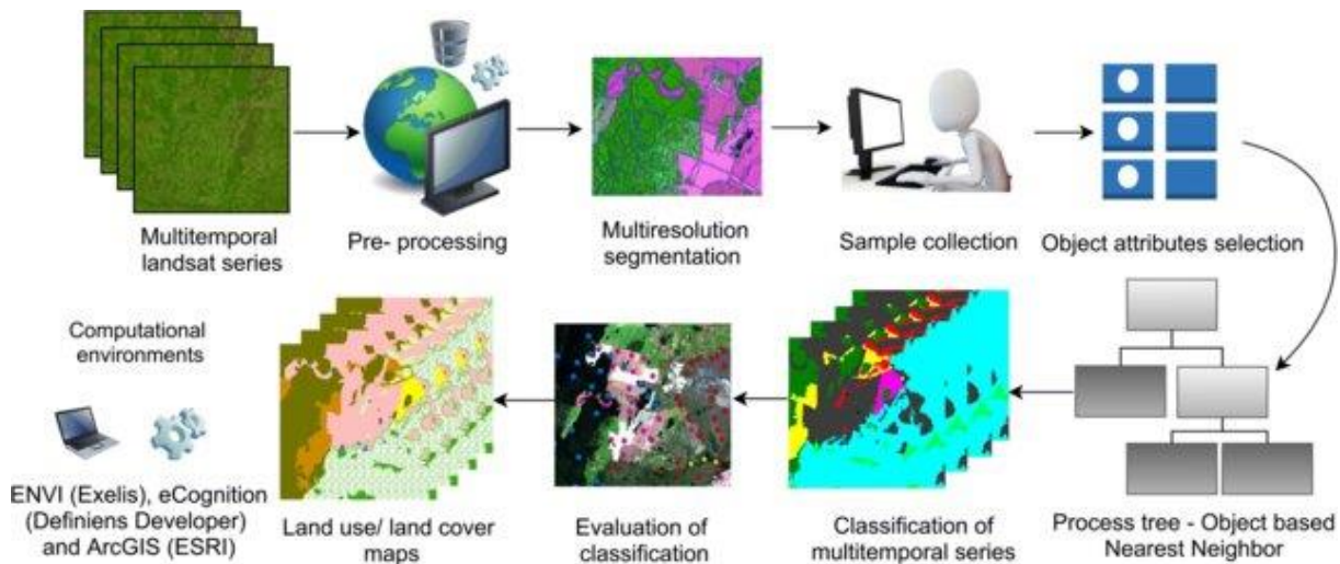
Figure N° 06 : Processus of Image Classification. Source : Da Cunha, E. R., et al 2020
