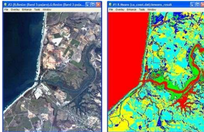
Figure N° 08 : Unsupervised Classification. Source : Da Cunha, E. R., et al 2020
